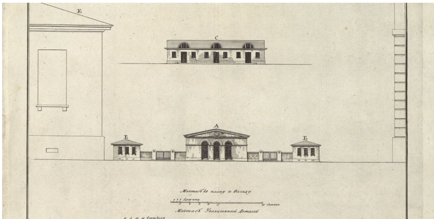
План и фасад станционного дома. 1824 г. Главархив Москвы. Фото: Главное архивное управление города Москвы
